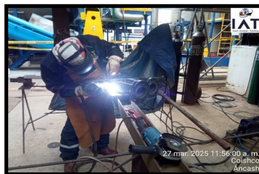
SOLDEO DE TUBERIA DE VAPOR
